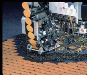
シークイン装置Ⅳ 小径から大径、異形や偏芯シークインを 刺繍する装置
